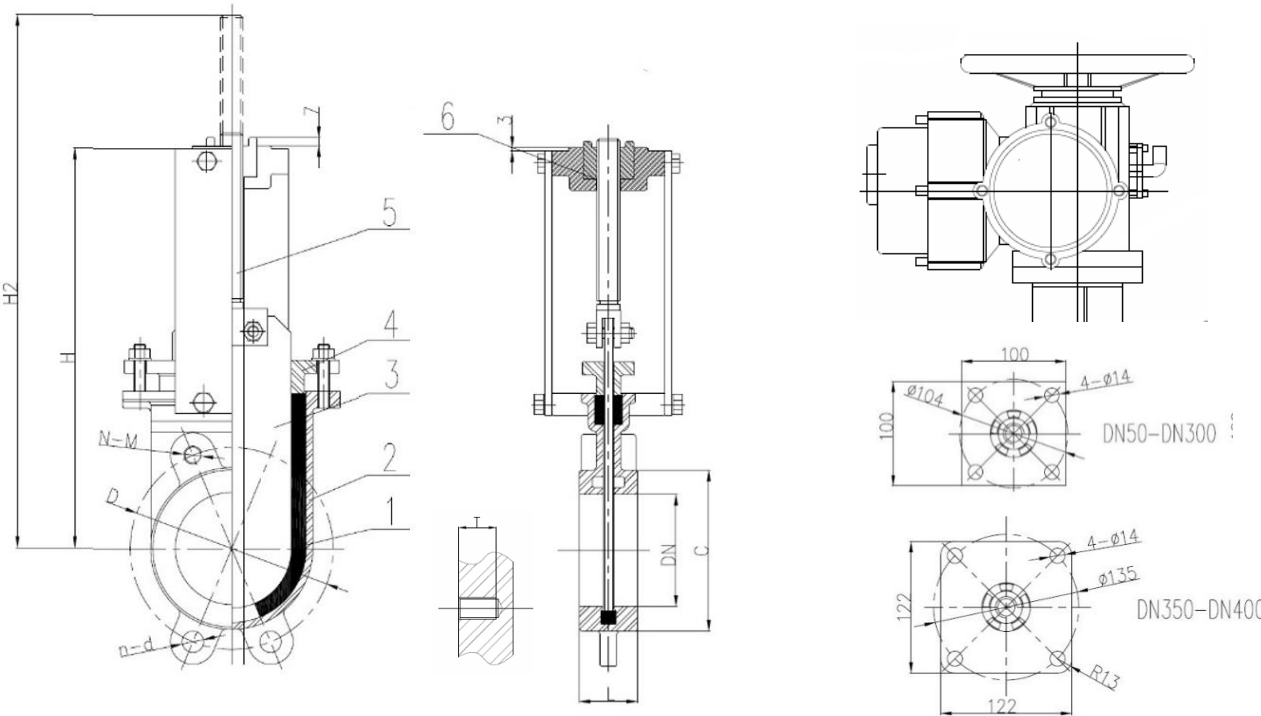
Рис. 1. Габаритные и присоединительные размеры шиберной задвижки.
