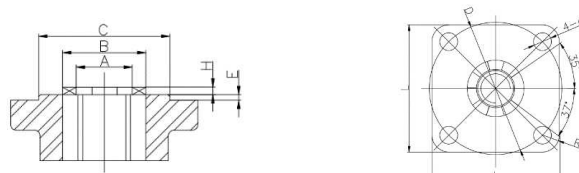
Рис. 2. Фланец шиберной задвижки под электропривод.
