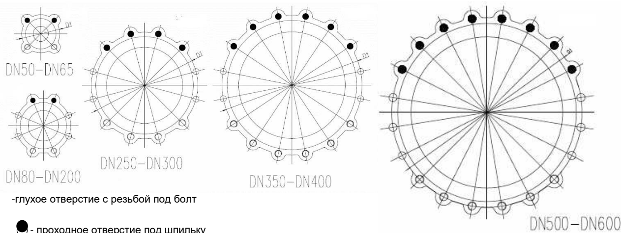
Рис. 3. Схема крепежных отверстий шиберных задвижек.
