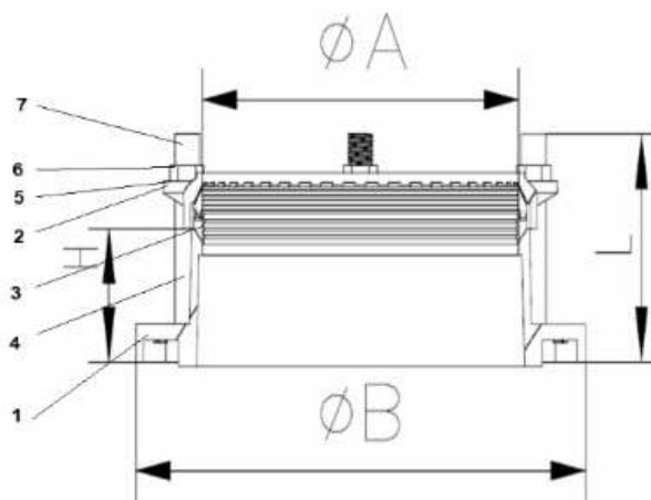
Рис.4. Муфта/адаптер ПФРК-Е.
