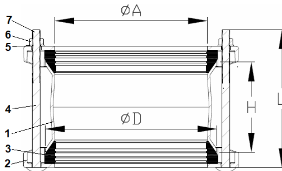
Рис.1. Муфта ДРК
