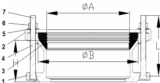
Рис.3. Муфта/адаптер ПФРК
