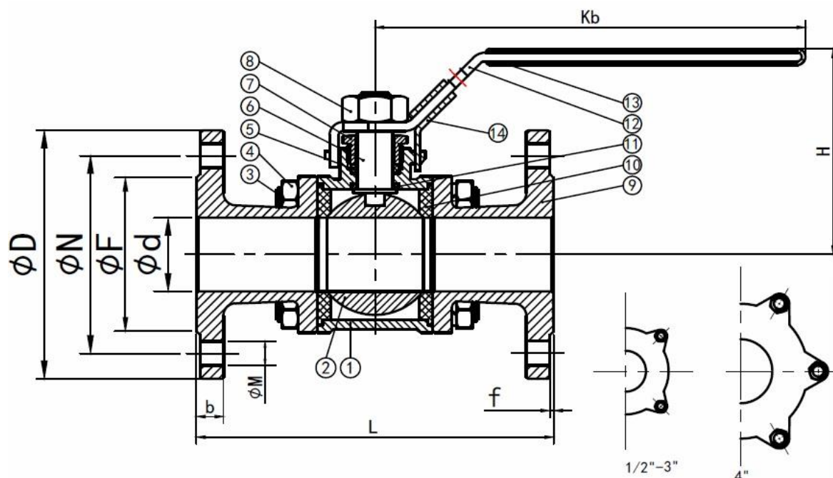
Рис.1 Кран трехсоставной шаровой фланцевый.
