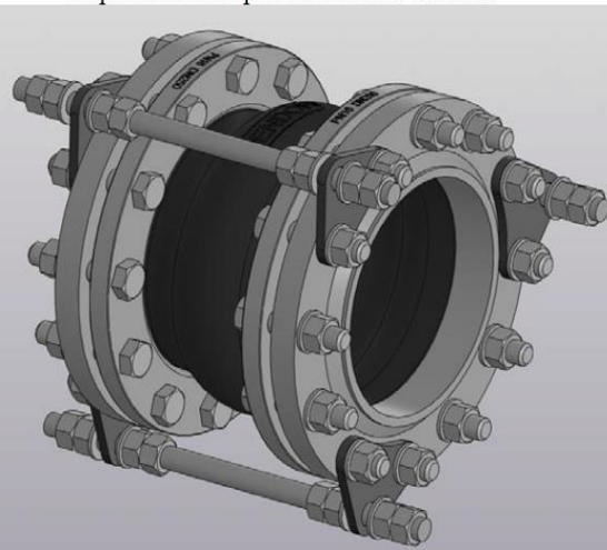
Ограничитель растяжения и сжатия
