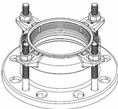
Рис.4. Муфта/адаптер ПФРК-Е.
