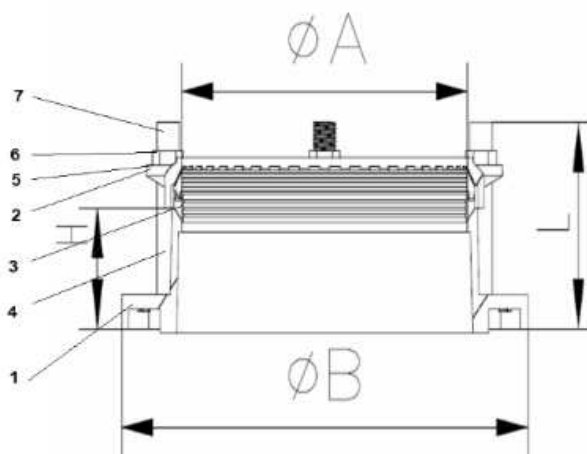
Рис.4. Муфта/адаптер ПФРК-Е.
