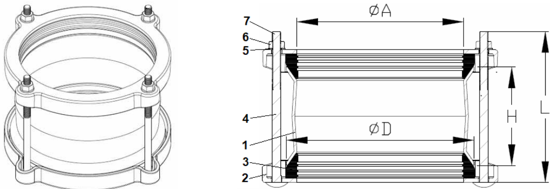
Рис.1. Муфта ДРК
