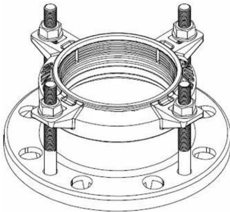
Рис.4. Муфта/адаптер ПФРК-Е.
