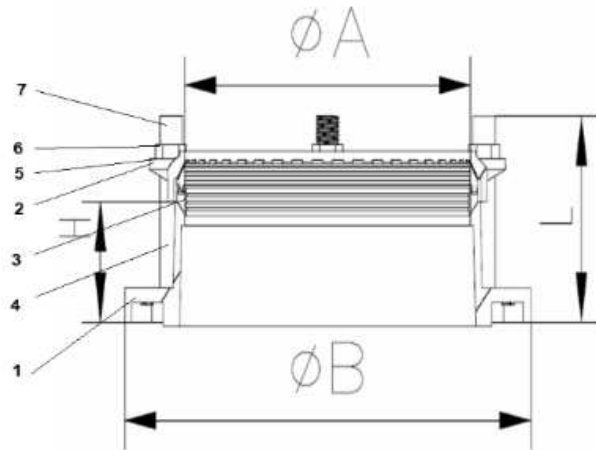
Рис.4. Муфта/адаптер ПФРК-Е.
