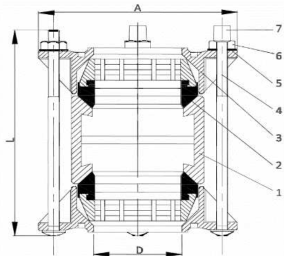
Рис.2. Муфта ДПК-Е
