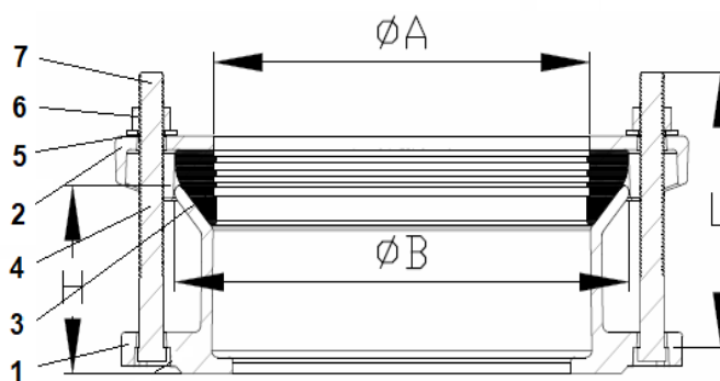
Рис.3. Муфта/адаптер ПФРК
