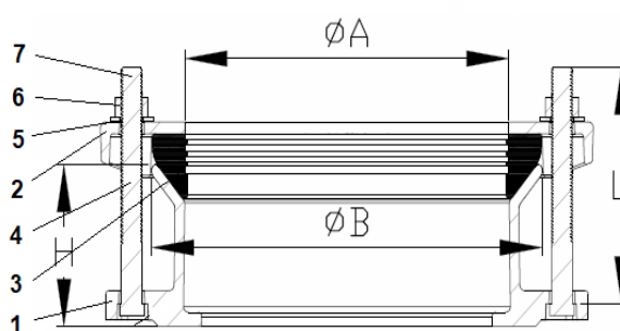
Рис.3. Муфта/адаптер ПФРК
