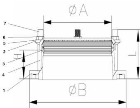
Рис.4. Муфта/адаптер ПФРК-Е
