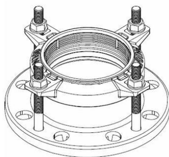
Рис.4. Муфта/адаптер ПФРК-Е
