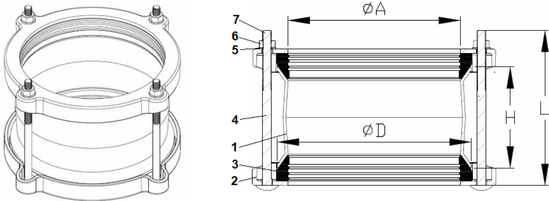
Рис.1. Муфта ДРК
