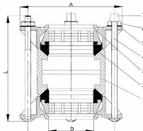
Рис.2. Муфта ДРК-Е
